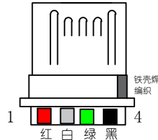
Micro usb公头焊接面
