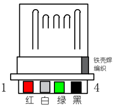
Micro usb公头焊接面
